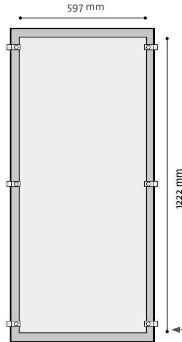
Ansicht D1300/D1000
