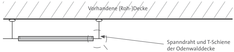
Ansicht D1300/D1000
